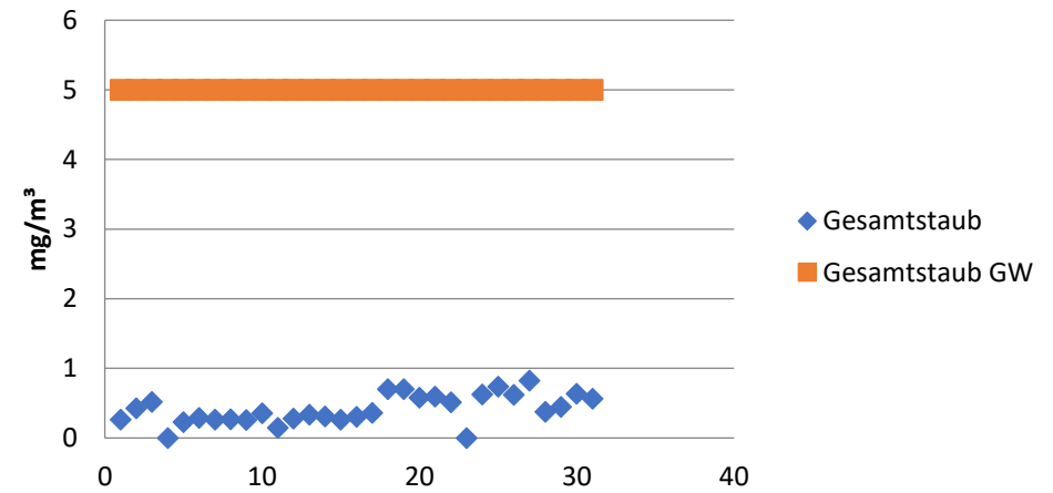
Gesamtstaub - Mai 2019
