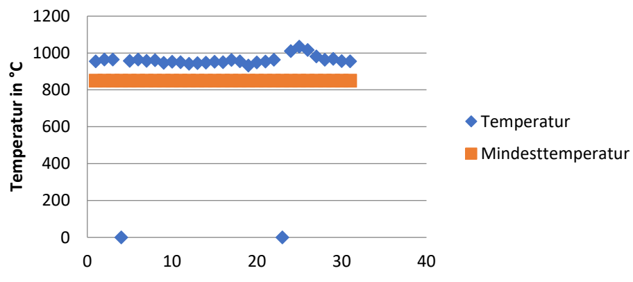
Verbrennungsbedingungen - Mai 2019
