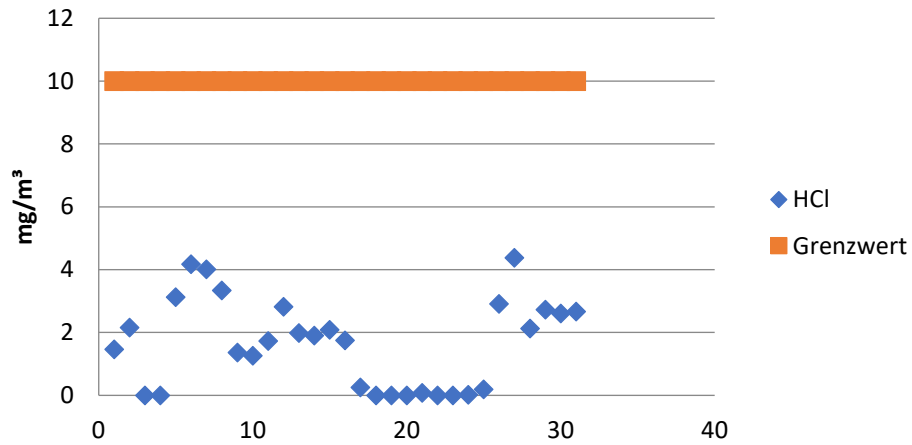
HCl - Mai 2019
