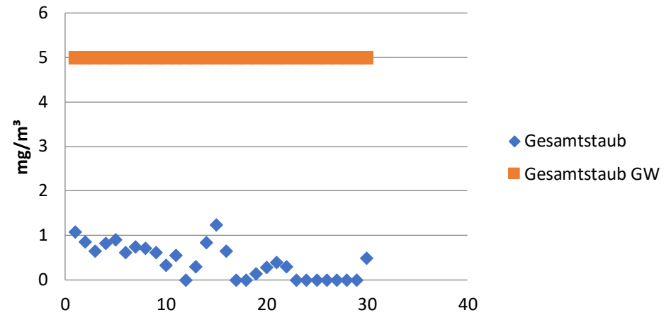
Gesamtstaub - April 2019
