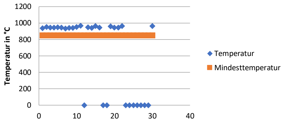
Verbrennungsbedingungen - April 2019
